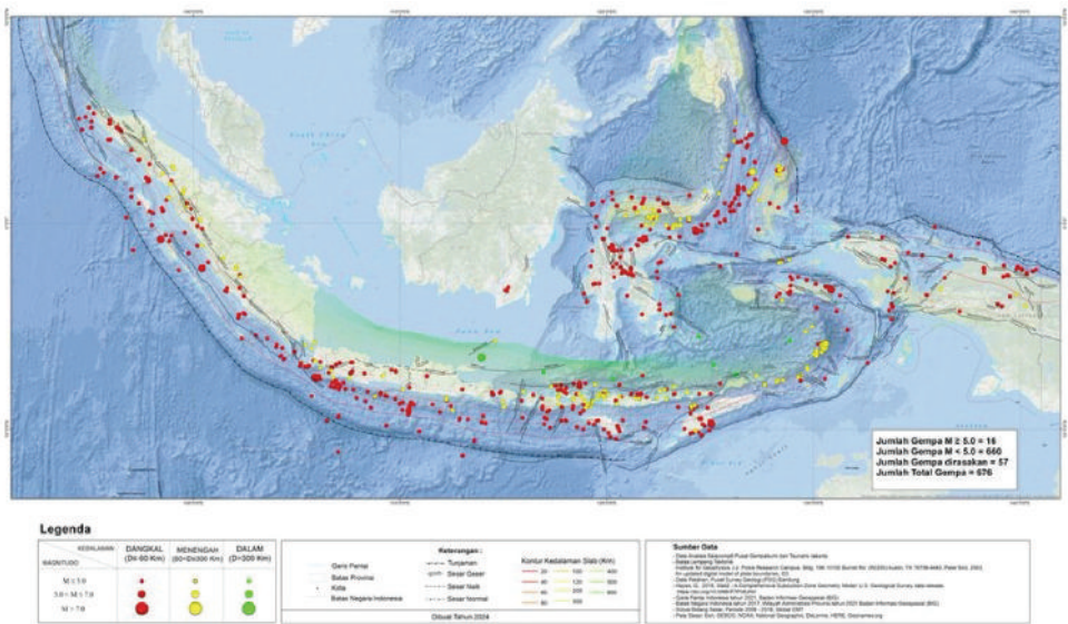
Gambar 2.3 Peta Seismisitas Indonesia Tahun 2024
